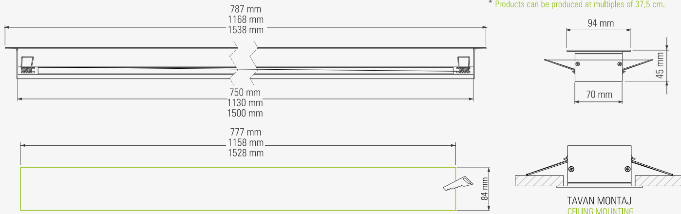
TAVAN KESİM ÖLÇÜSÜ CEILING CUT-OUT SIZE
